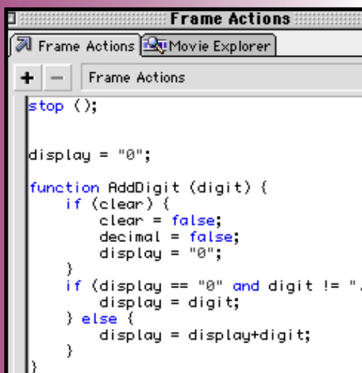
以判定語句設計計算機
